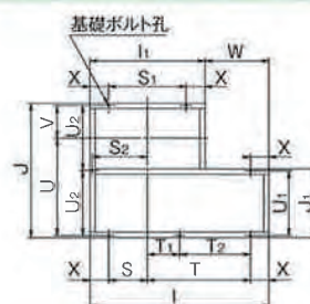
TH-L-D,TV-L-D, BH-R-D型用ベース
