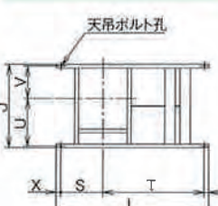
TH-L-G, TV-L-G, BH-R-G型用ベース
