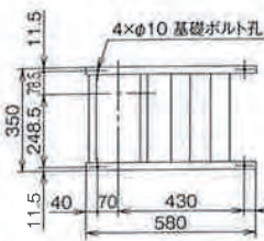
TH-R-I/G,TV-R-I/G,BH-L-I/G型用ベース
