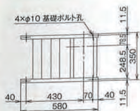
TH-R-I/G,TV-R-I/G,BH-L-I/G型用ベース
