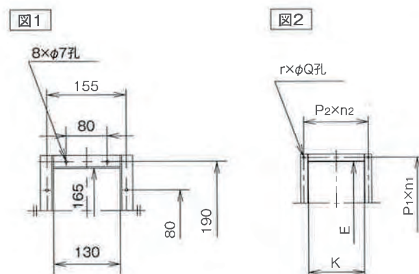
吐出相フランジ
