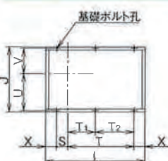
TH-L-G, TV-L-G, BH-R-G型用ベース
