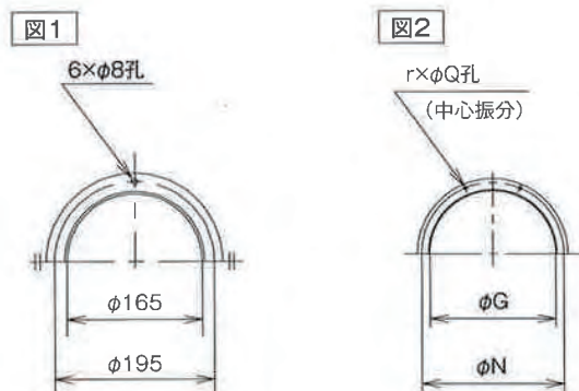
吸込相フランジ
