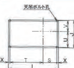
TH-R-I, TV-R-I, BH-L-I型用ベース
