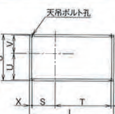
TH-L-I, TV-L-I, BH-R-I型用ベース
