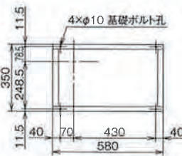
TH-L-I/G,TV-L-I/G,BH-R-I/G型用ベース
