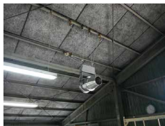
場内換気促進用 誘引ファン
