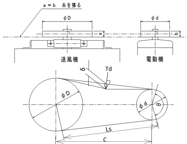
図1 芯出し
